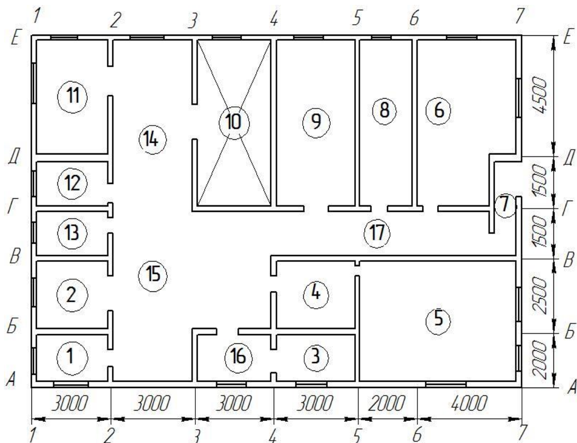
Рисунок 1 –План здания
