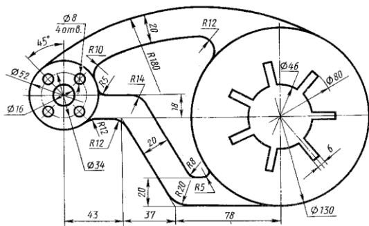
Опора
