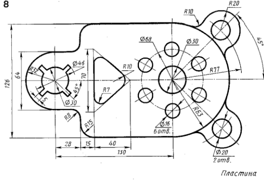
Пластина
