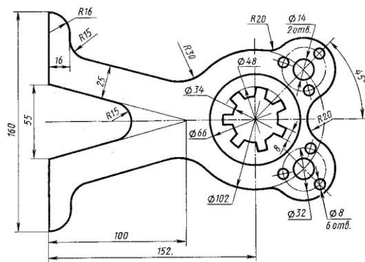
Кронштейн
